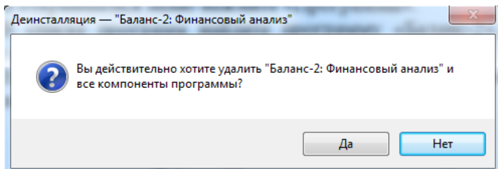
Рис.8 Окно деинсталляции
